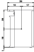
Seitenansicht
